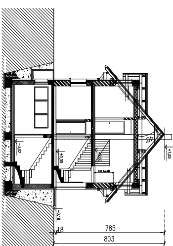
PREČNI PREREZ
