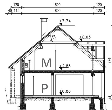
PREČNI PREREZ
