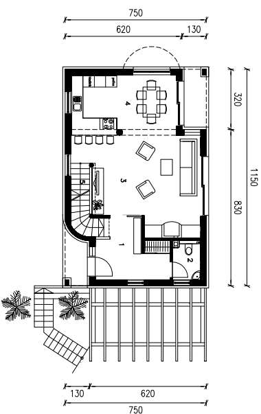
TLORIS PRITLIČJA M=1:200
