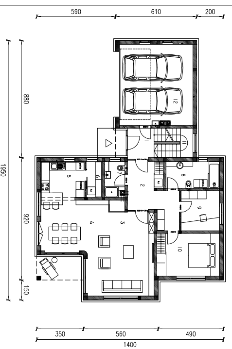
TLORIS PRITLIČJA M=1:200
