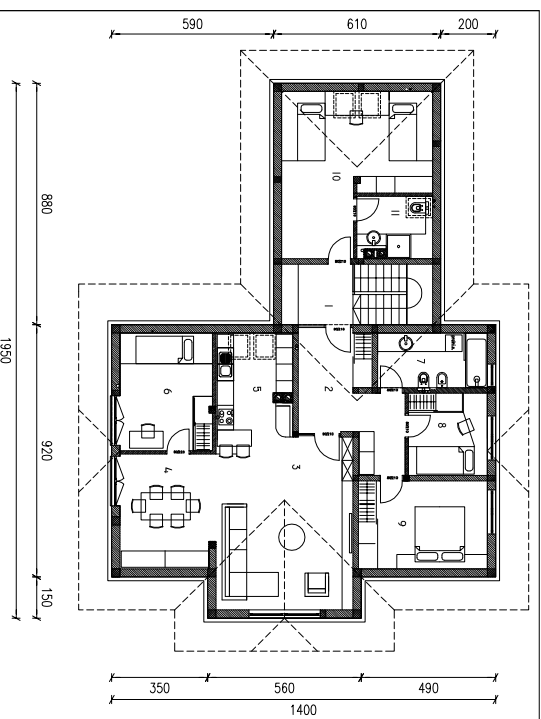
TLORIS MANSARDE M=1:200
